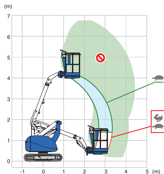
AA-9MC Arbeitsbereich
