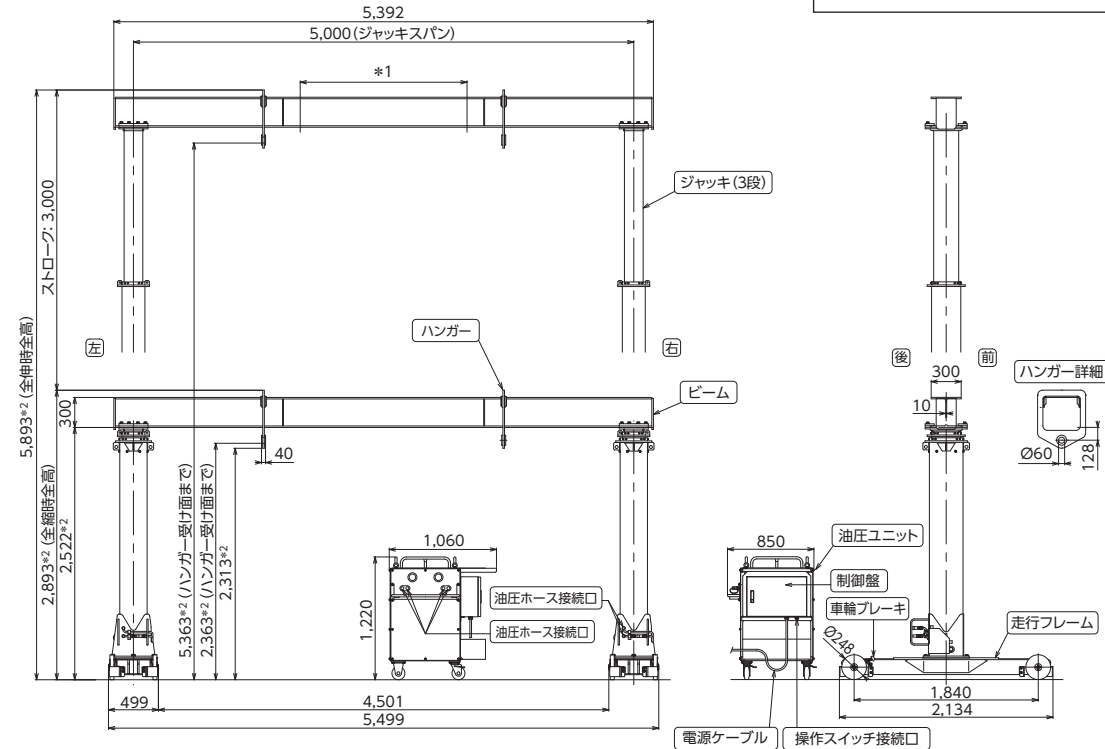
外観図 (単位: mm)
