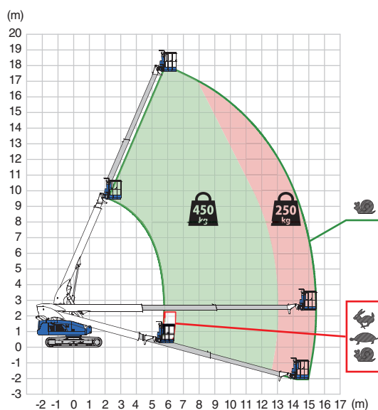
Werkbereik AS-20MC
